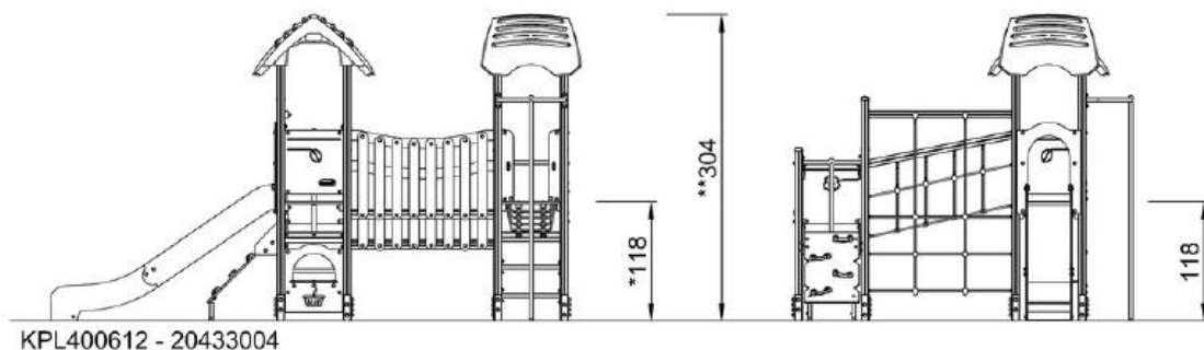
Figur 3. opstalttegning.
